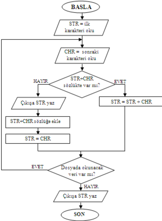
Şekil 4.6. Lzw Sıkıştırma Algoritması
