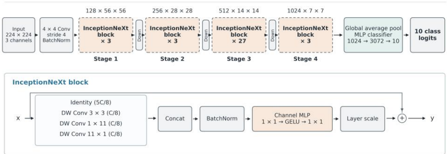
InceptionNeXt-Base
