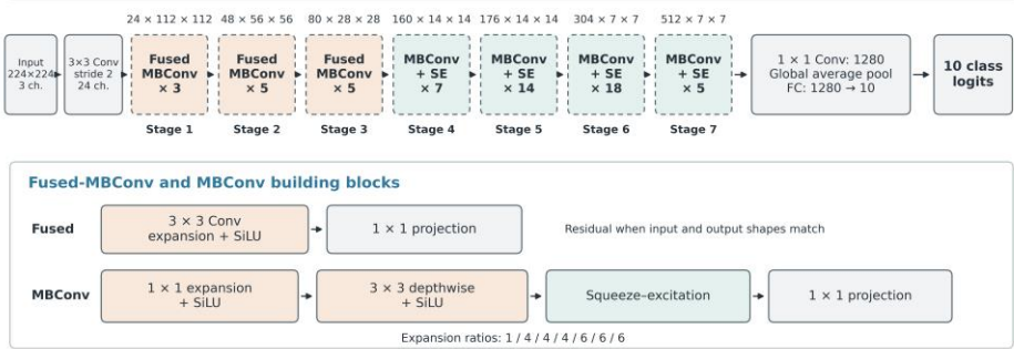
EfficientNetV2-M
