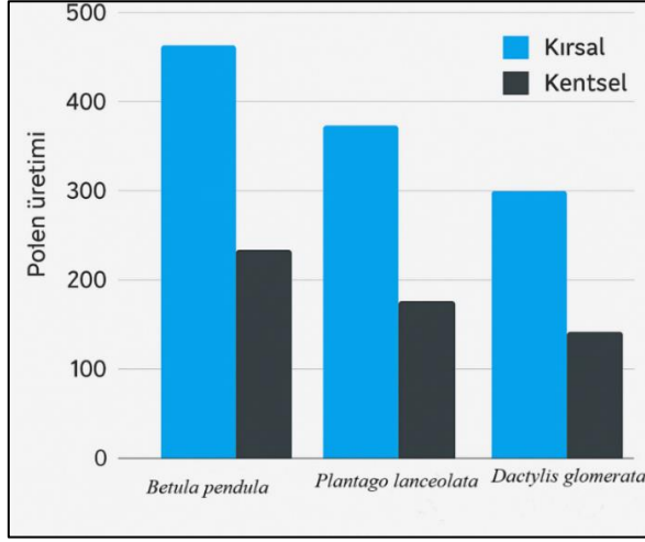
Şekil 4: Betula pendula (huş), Plantago lanceolata ve Dactylis glomerata bitkilerinin polen üretim miktarının kırsal ve kentsel alanlardaki değişimi.
