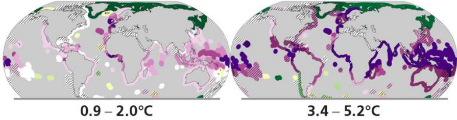
Şekil 6. Balıkçılık ile İlgili Sıcaklık Artışı Projeksiyonu (Kaynak: IPCC, 2023)
