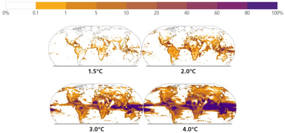
Şekil 3. Sıcaklığa Bağlı Tür Kayıpları Risk Haritası (Kaynak: IPCC, 2023)
