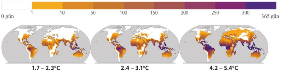
Şekil 4. İnsan Sağlığı için Isı ve Nem Riski (Kaynak: IPCC, 2023)
