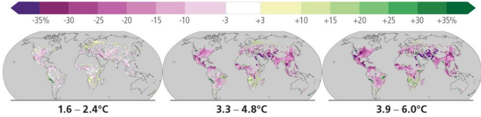
Şekil 5. Mısır Verimi ile İlgili Sıcaklık Artışı Projeksiyonu (Kaynak: IPCC, 2023)
