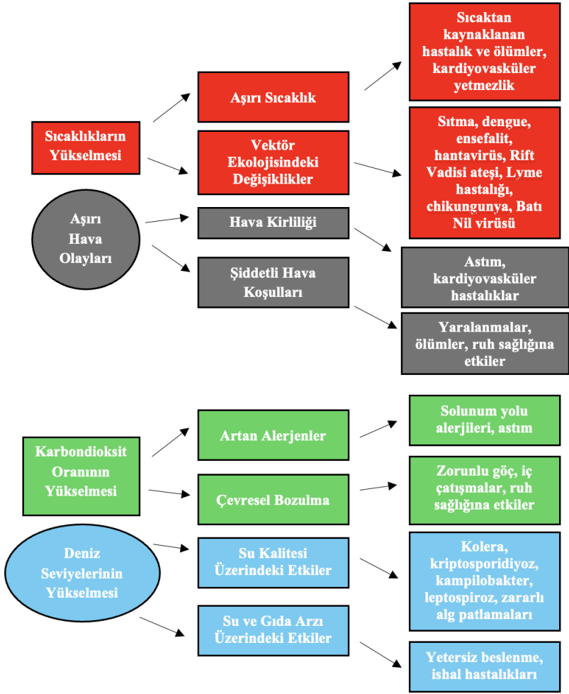
Şekil 1. Küresel Isınmanın Olası Biyo-Psiko-Sosyal Etkileri (Kaynak: McCarty ve ark., 2009)
