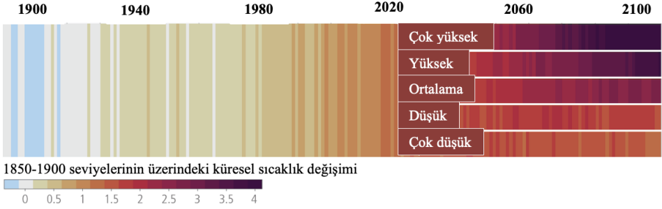
Şekil 2. Küresel Isınma ile ilgili Geçmiş Durum ve Gelecek Projeksiyonu (Kaynak: IPCC, 2023)
