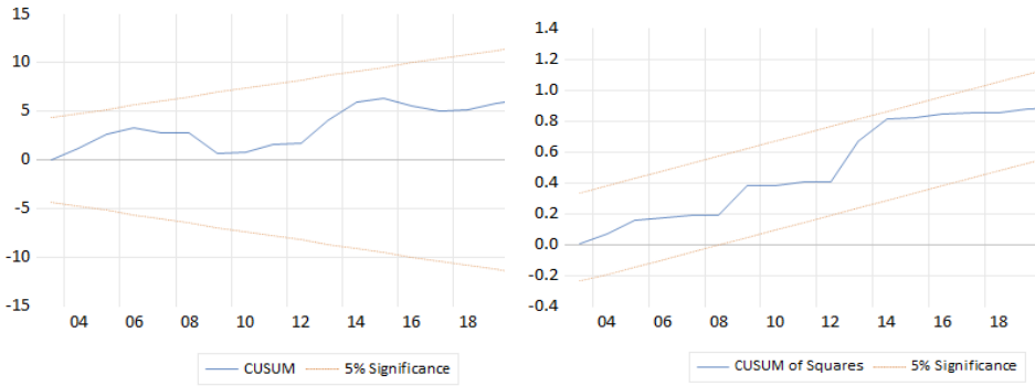
Şekil 1. CUSUM 7 ve CUSUMSQ 8 Testleri Bulguları
